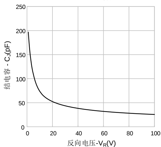
图 3. 结电容特性
