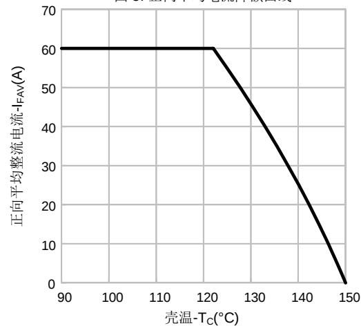
图 5. 正向平均电流降额曲线
