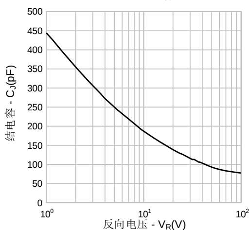
图 4. 结电容特性
