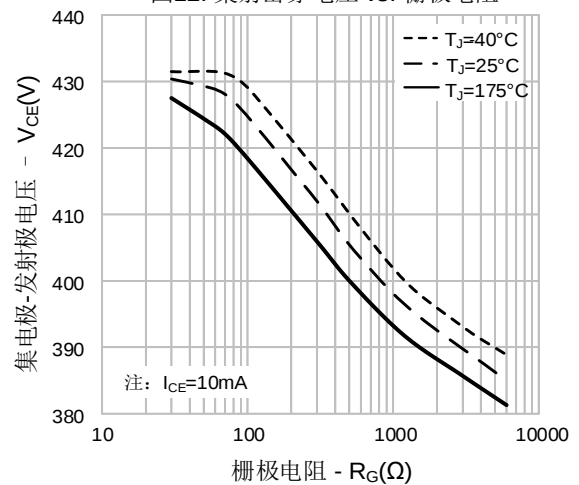
图12. 集射击穿电压 vs. 栅极电阻
