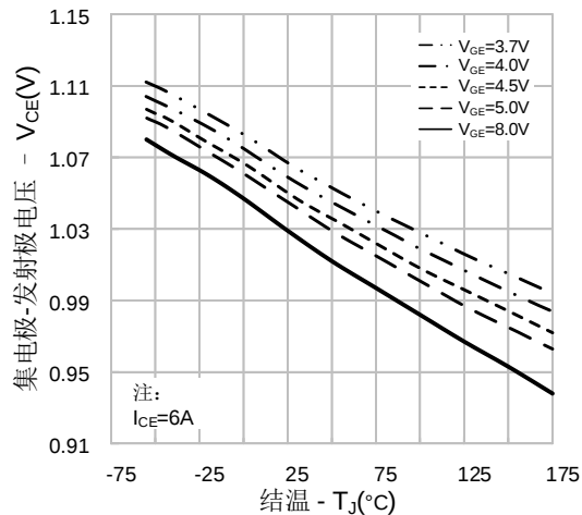
图5. 饱和电压 vs. 温度
