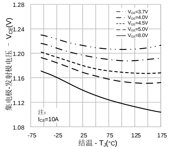
图6. 饱和电压 vs. 温度
