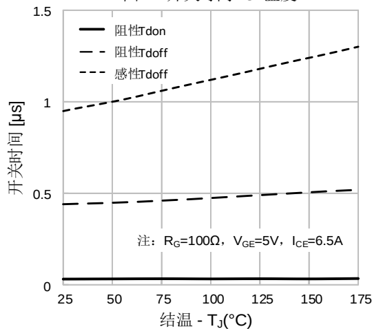
图11. 开关时间 vs. 温度
