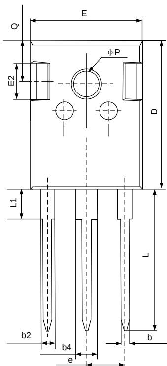
TO-247-3L
