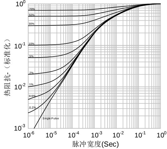
图21. 二极管瞬态热阻抗 vs. 脉冲宽度
