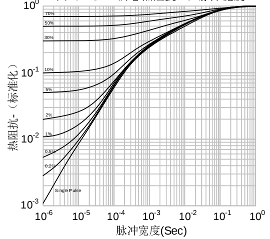
图20. IGBT 瞬态热阻抗 vs. 脉冲宽度
