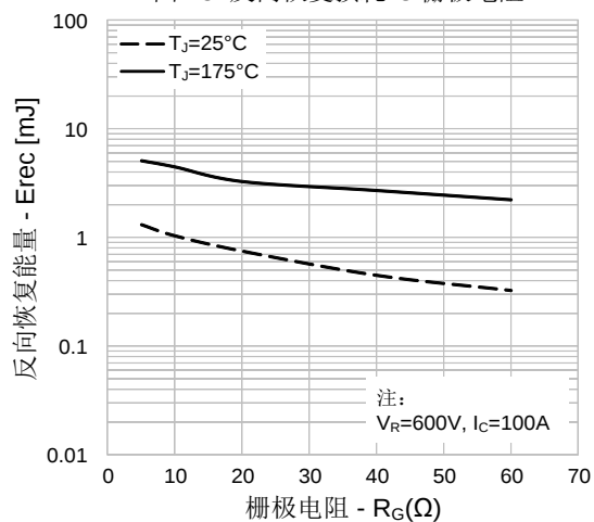
图 28. 反向恢复损耗 vs. 栅极电阻
