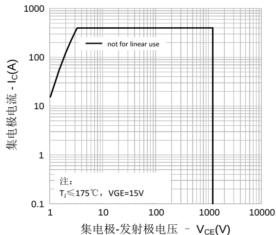
图 30. 安全工作区
