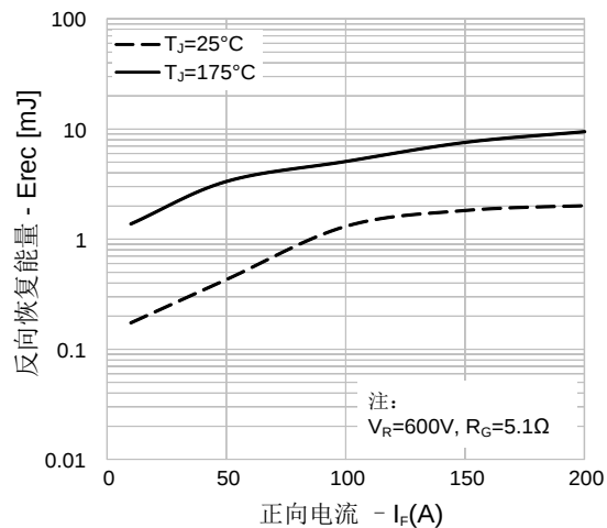
图29. 反向恢复损耗 vs. 正向电流
