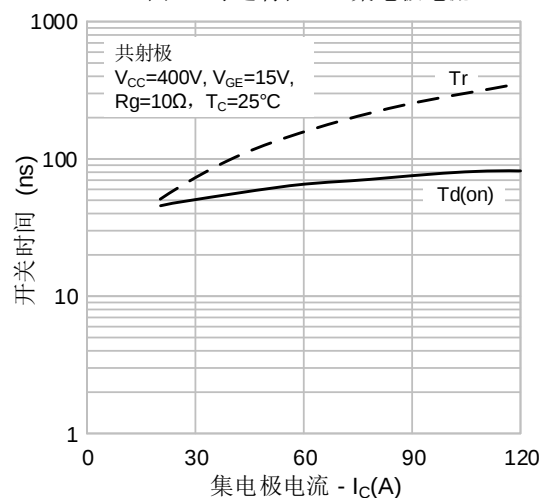
图12. 导通特性 vs. 集电极电流
