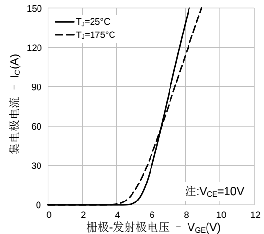
图4. 传输特性
