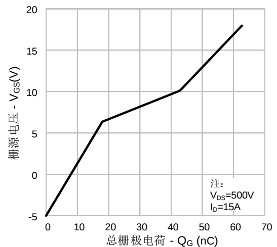
图 12. 电荷量特性
