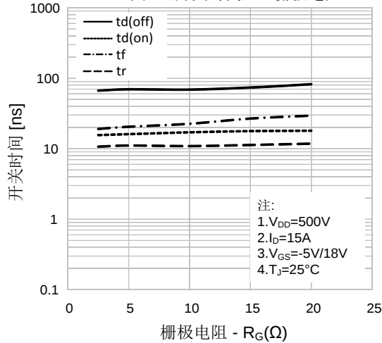
图23. 开关时间 vs. 栅极电阻
