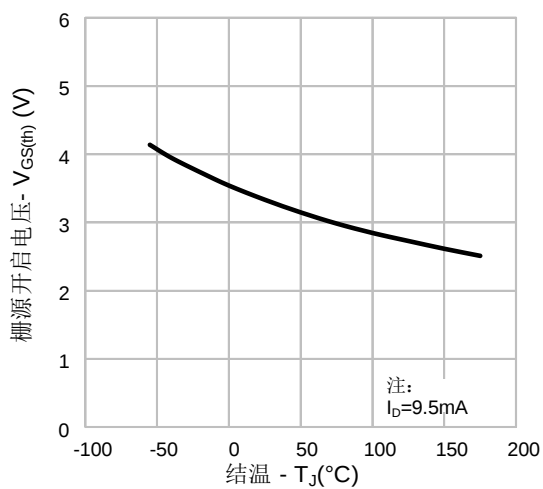
图 11. 开启电压 vs. 温度特性
