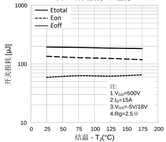
图22. 开关损耗 vs. 温度
