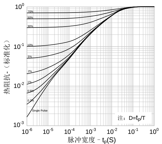
图18.瞬态热阻抗 vs. 脉冲宽度
