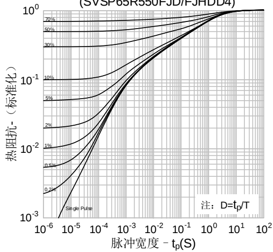
图16-2.瞬态热阻抗 vs. 脉冲宽度 (SVSP65R550FJD/FJHDD4)
