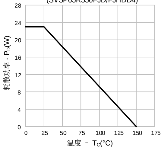
图14-2. 耗散功率vs.温度 (SVSP65R550FJD/FJHDD4)
