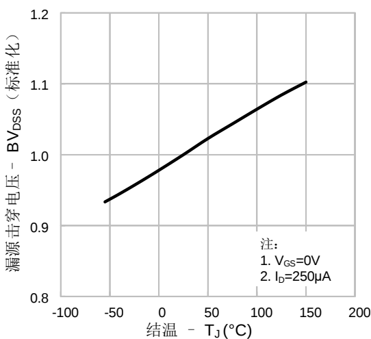
图 11. 击穿电压 vs. 温度特性
