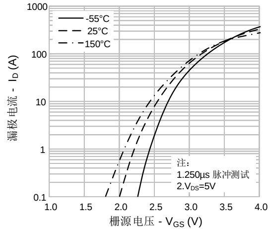
图 2. 传输特性
