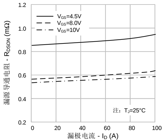
图 3. 导通电阻 vs. 漏极电流
