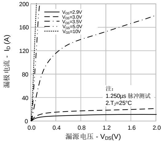
图 1. 输出特性
