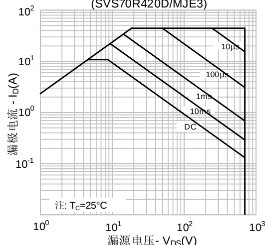
图 12-1. 最大安全工作区域 (SVS70R420D/MJE3)
