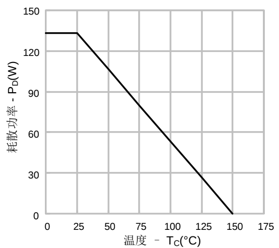
图14-3. 耗散功率vs.温度(SVS65R280T/SD4)
