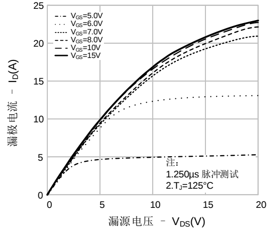
图 2. 输出特性
