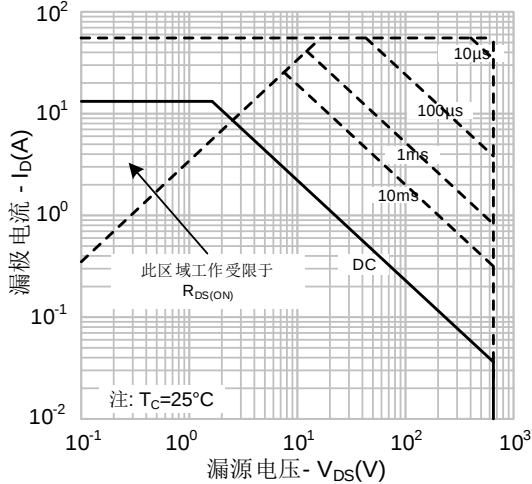
图 13-3. 最大安全工作区域(SVS65R280T/SD4)
