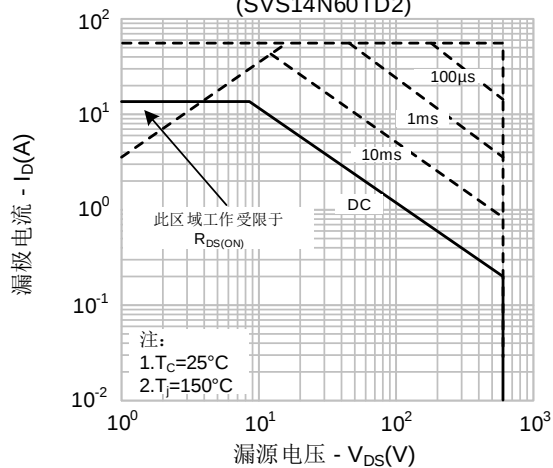
图9-1. 最大安全工作区域 (SVS14N60TD2)
