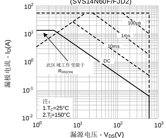
图9-2. 最大安全工作区域 (SVS14N60F/FJD2)
