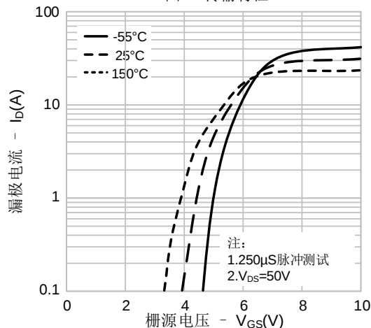
图 2. 传输特性
