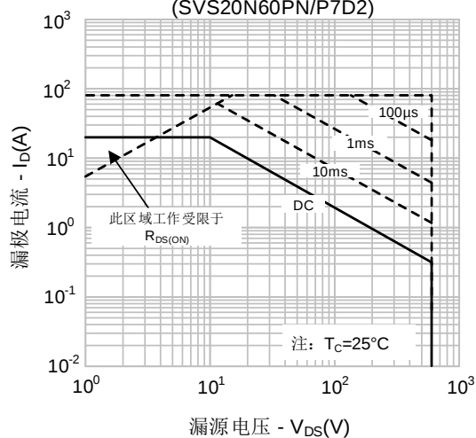
图9-3. 最大安全工作区域 (SVS20N60PN/P7D2)
