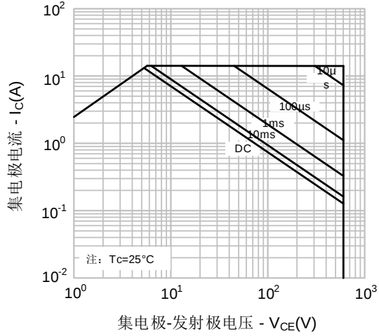
图21. 最大安全工作区域(SGTP5T60SD1S)
