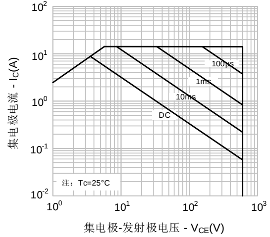
图20. 最大安全工作区域(SGTP5T60SD1F)
