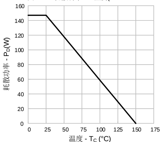
图 13-3. 耗散功率VS.温度(SVS70R360DE3)
