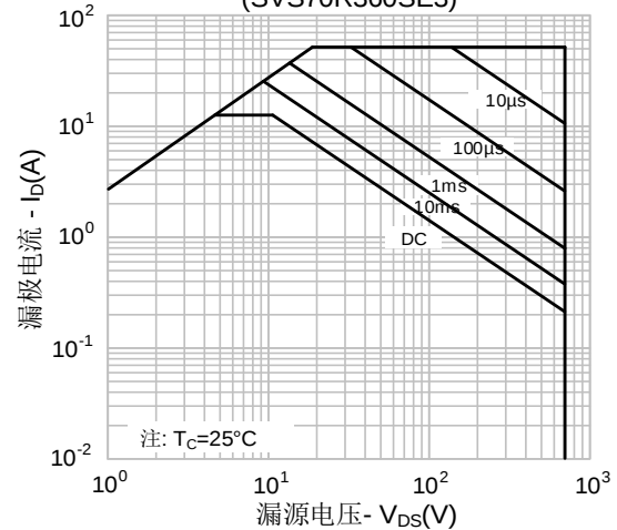
图 12-1. 最大安全工作区域 (SVS70R360SE3)
