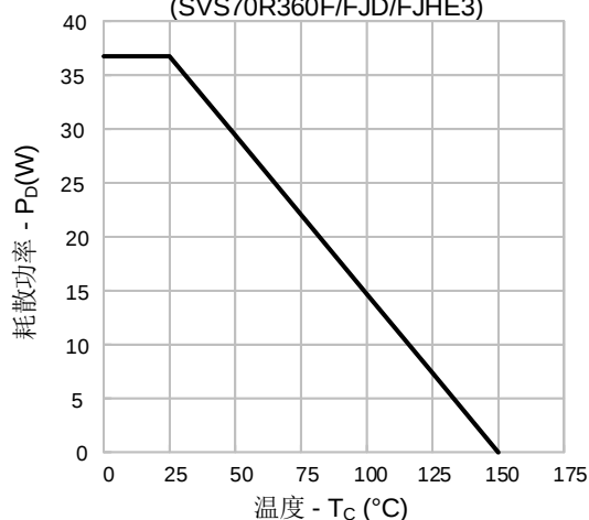
图 13-2. 耗散功率VS.温度 (SVS70R360F/FJD/FJHE3)
