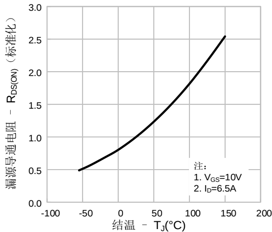
图 11. 导通电阻vs.温度特性
