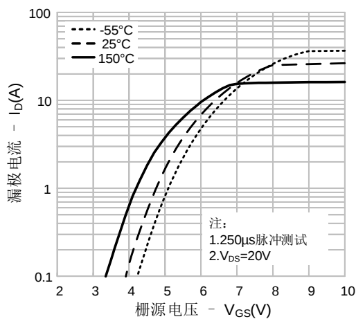
图 3. 传输特性
