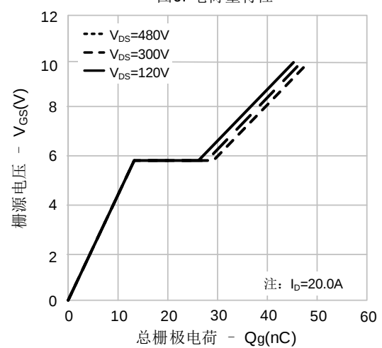
图6. 电荷量特性
