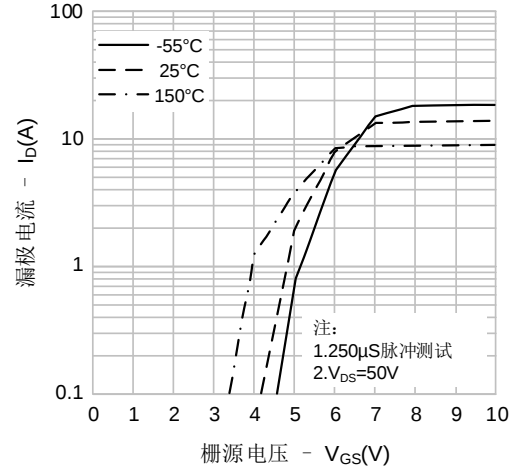
图2. 传输特性
