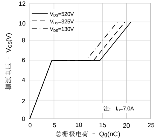
图6. 电荷量特性
