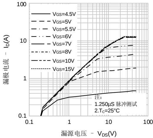
图1. 输出特性
