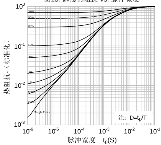
图15. 瞬态热阻抗 vs. 脉冲宽度
