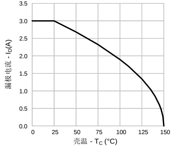
图 14. 漏极电流 vs. 壳温
