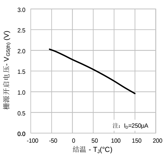
图 5. 开启电压 vs. 温度特性
