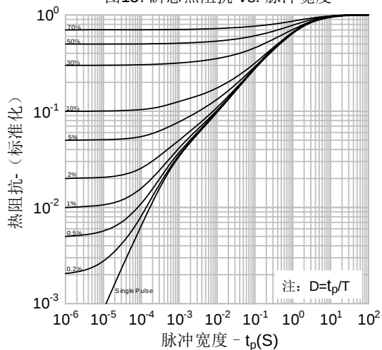
图15. 瞬态热阻抗 vs. 脉冲宽度
