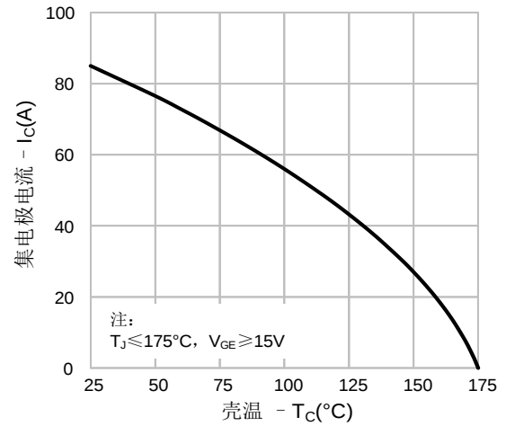
图26. 集电极电流 vs. 壳温
