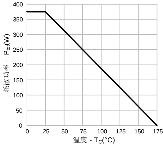
图 25. 耗散功率 vs. 温度
