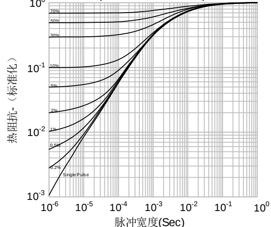
图42. 二极管瞬态热阻抗vs.脉冲宽度 (SGTP15U65SDM1S)
