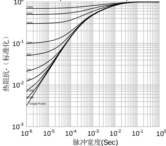
图41. IGBT 瞬态热阻抗vs.脉冲宽度 (SGTP15U65SDM1S)
